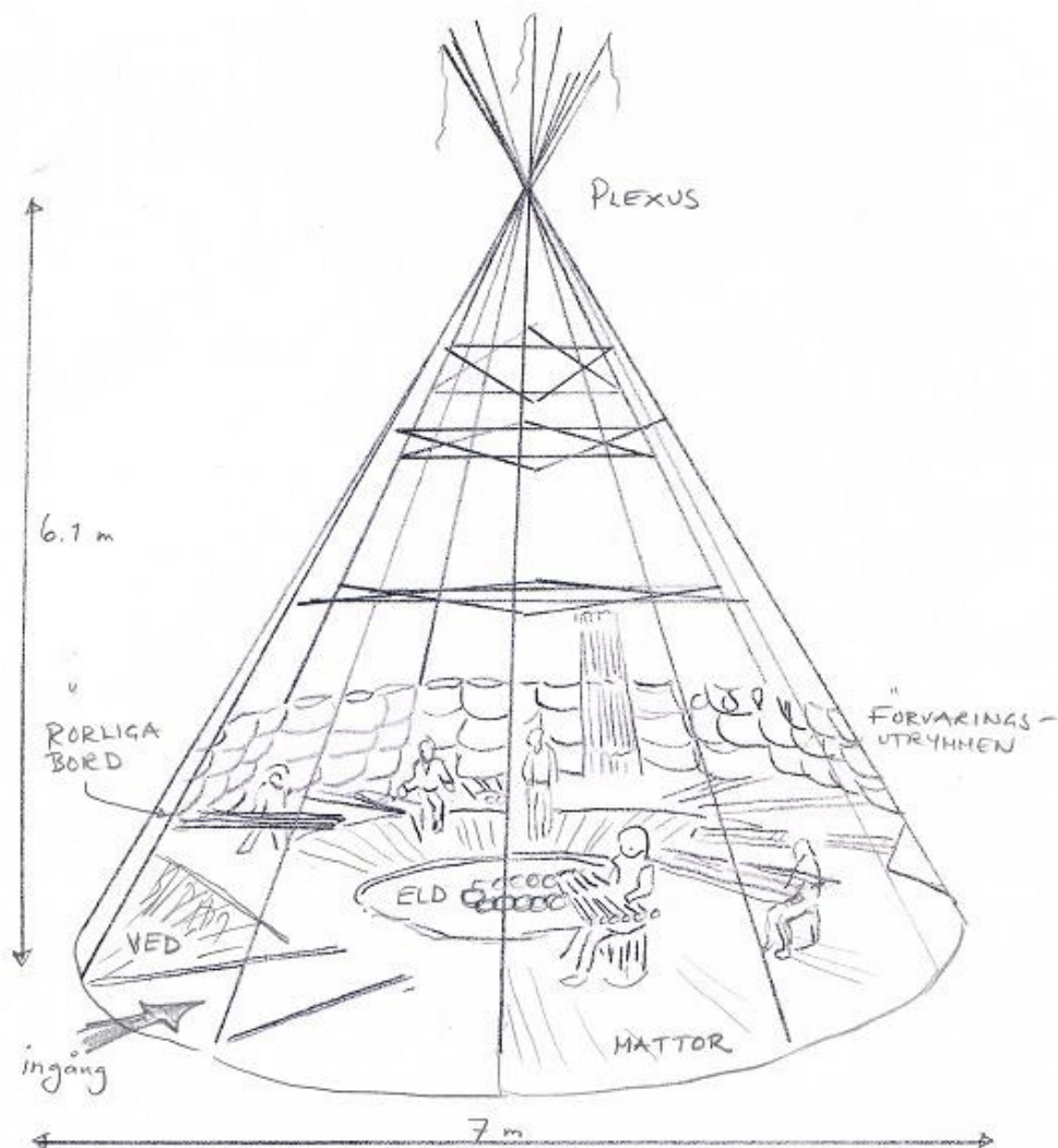
Figur 2 – En gwam - Detta är den matematiska principen för 7 meters gwamens uppbyggnad. Eldstaden är en meter i diameter. Utrymmet i ytterkanten där ligg- och sittplatser är placerade är två meter, gången mellan detta utrymme och eldstaden är en meter bred.
