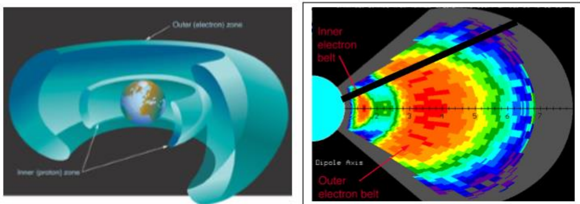
Van Allen-bältena 9
